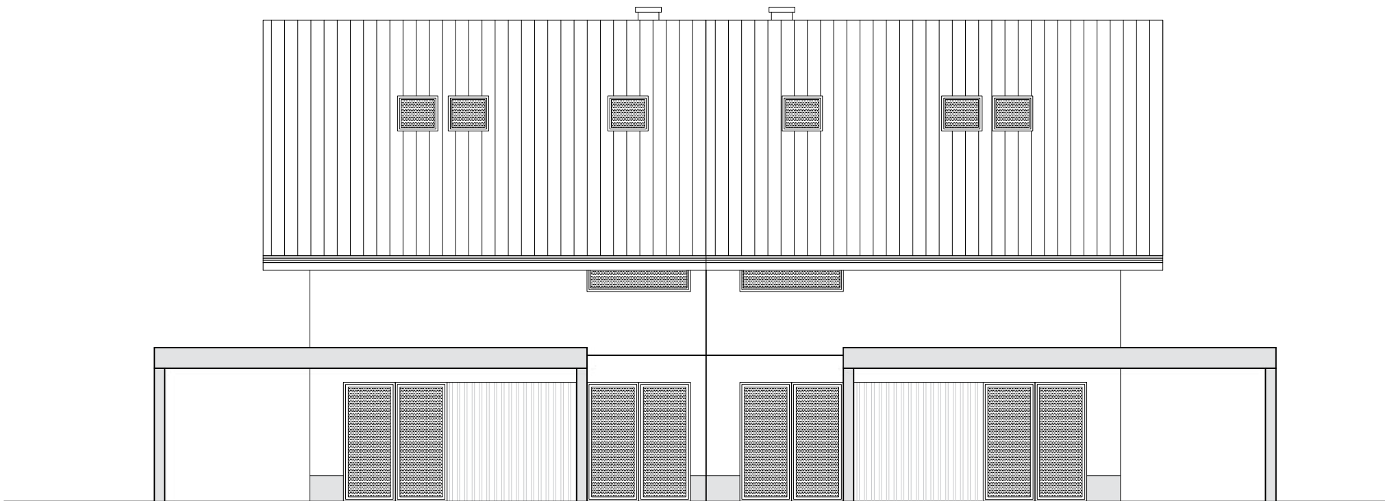
ZAHODNA FASADA
