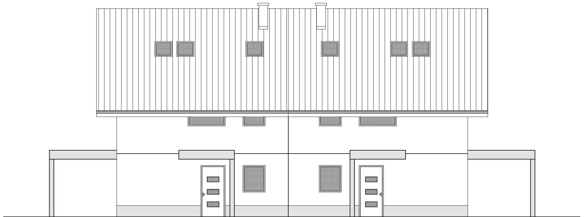
VZHODNA FASADA
